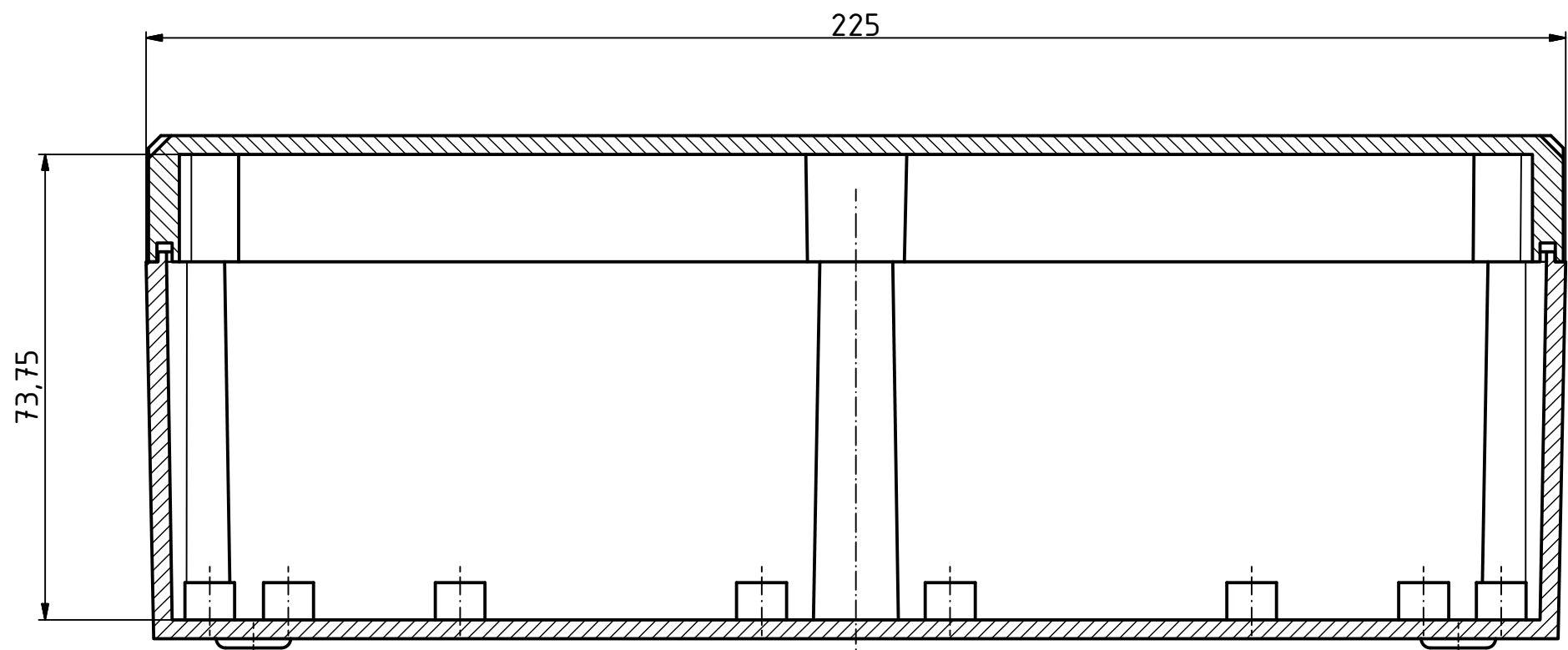
A-A ( 1 : 1 )
