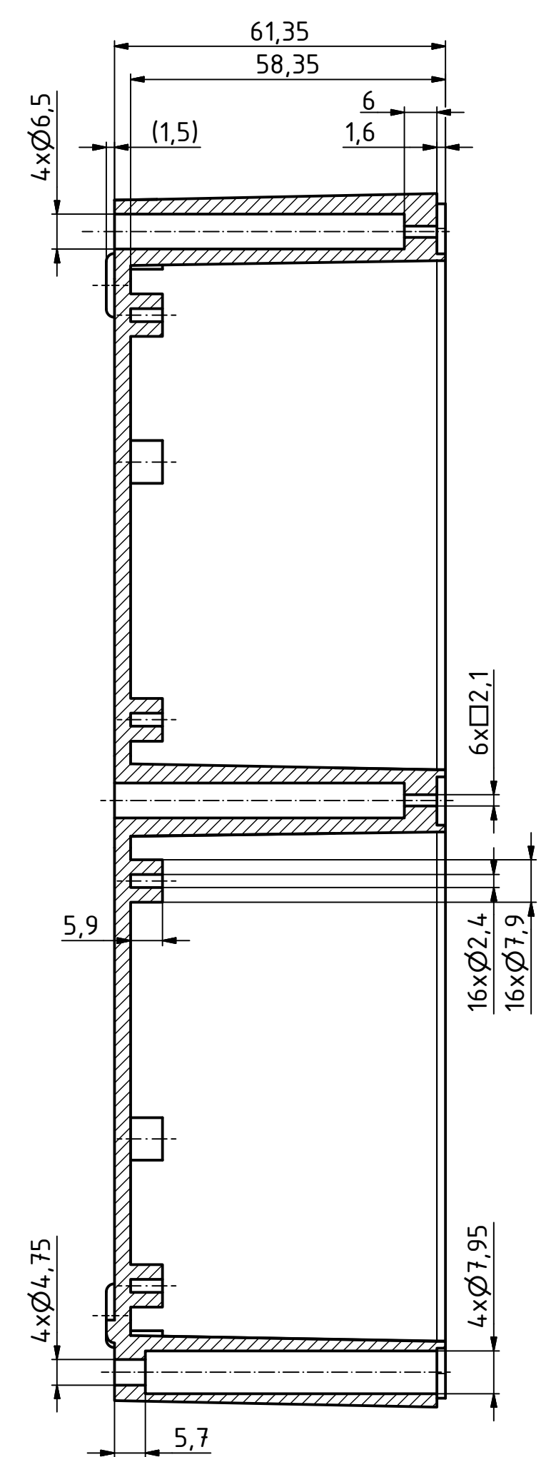
B-B ( 1 : 1 )
