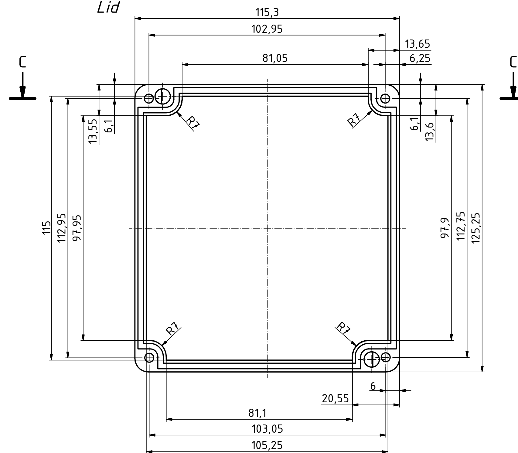
Oberteil/ Lid
