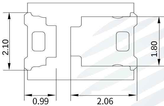
Fig.1-3 Bottom view 背面视图
