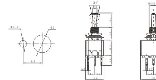
MTS-302-A2 ON-ON MTS-303-A2 ON-OFF-ON 3PDT 9P
