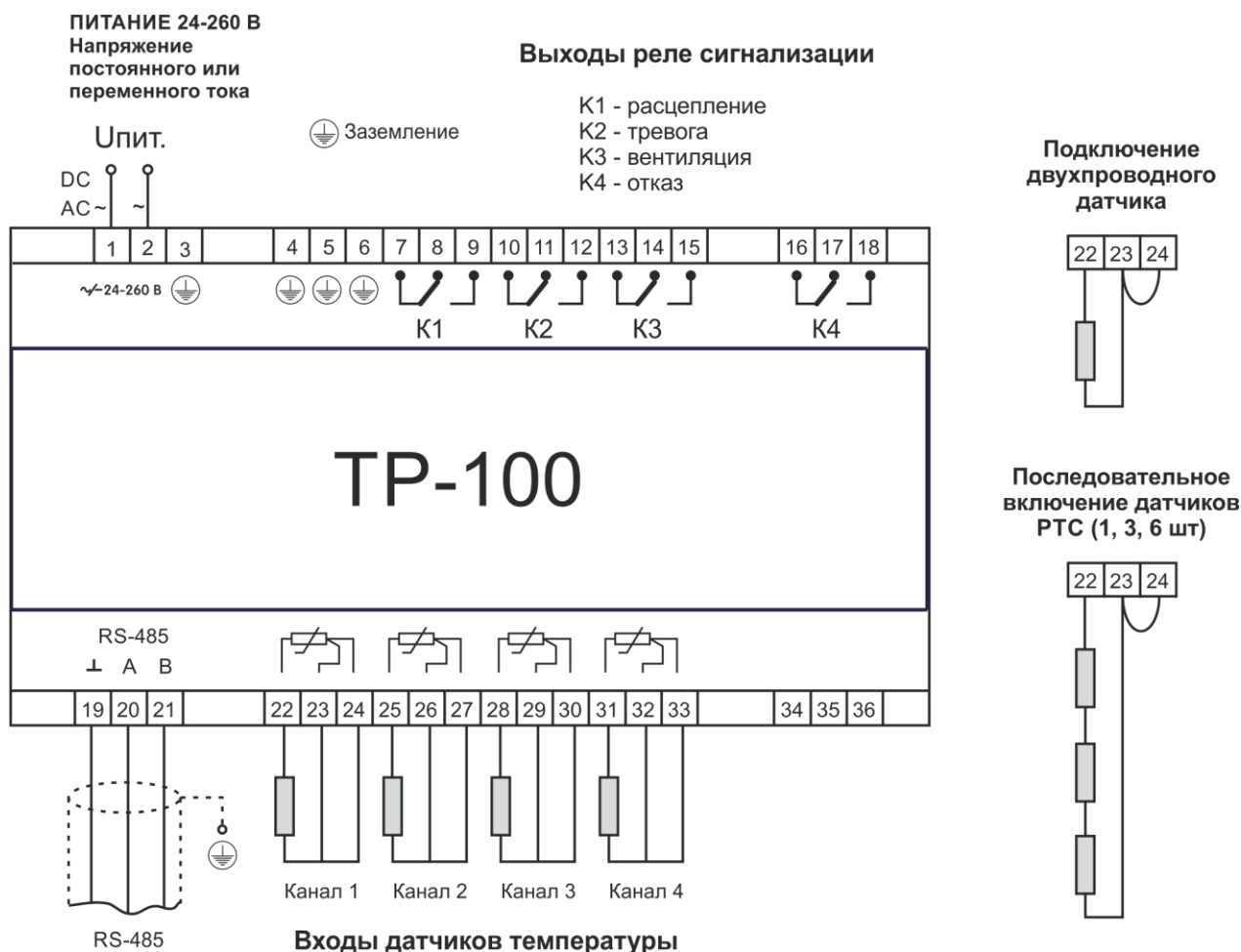
Рисунок 2 – Электрические соединения ТР-100
