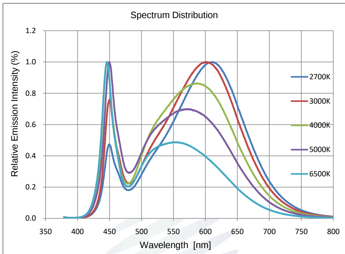
Fig 1-13 Spectrum Distribution 光谱分布特性曲线
