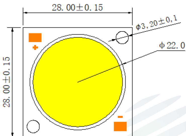
Fig.1-1 Top view 正面视图
