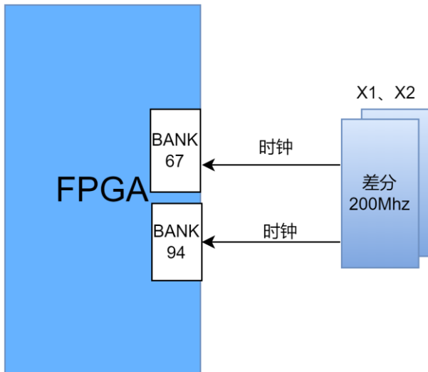
Figure 7: SOM module Clock Source
