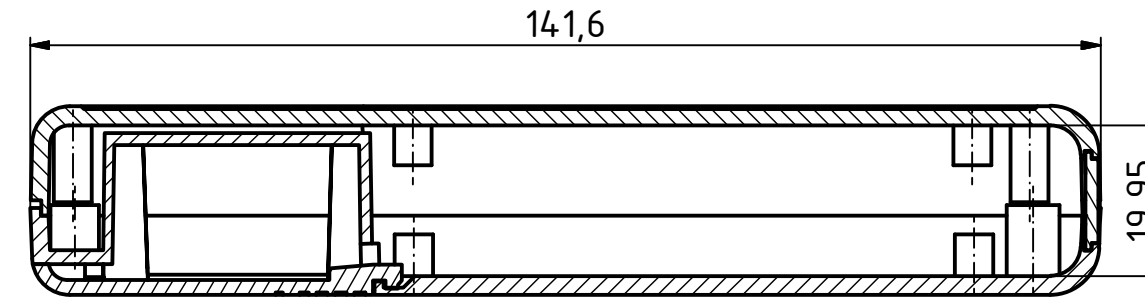
A-A ( 1 : 1 )
