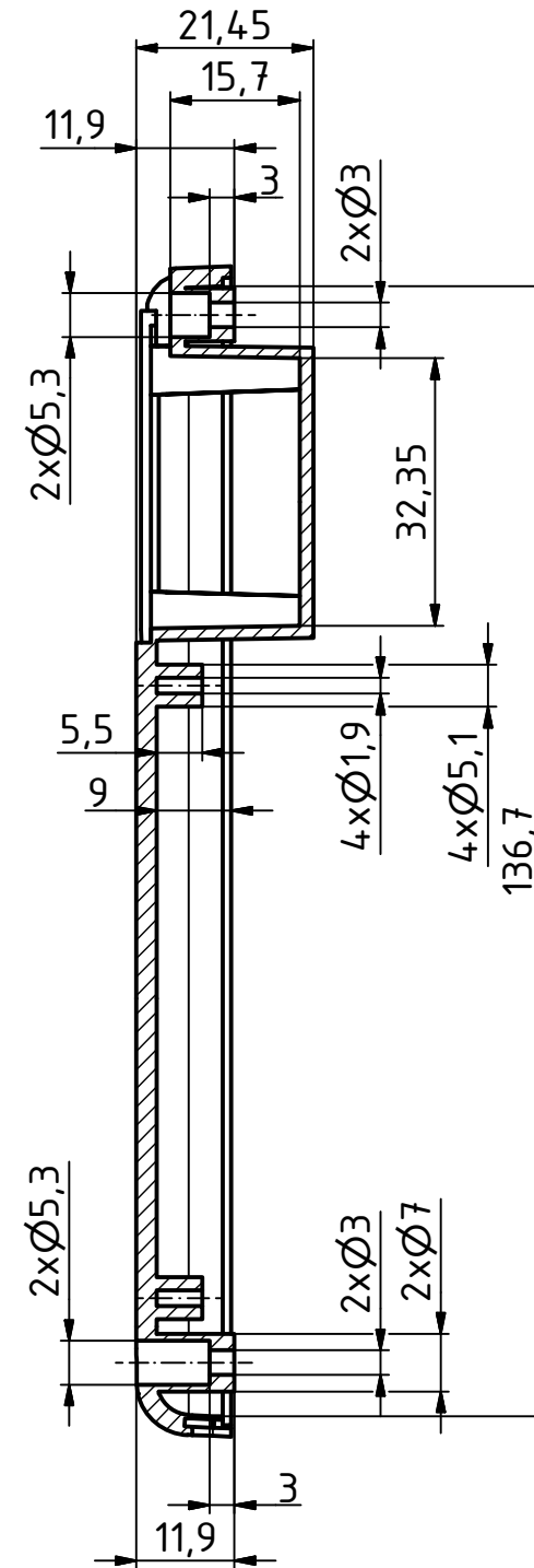
B-B ( 1 : 1 )
