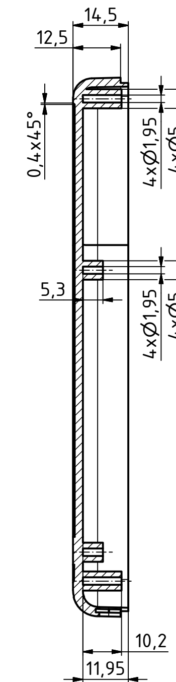
C-C ( 1 : 1 )
