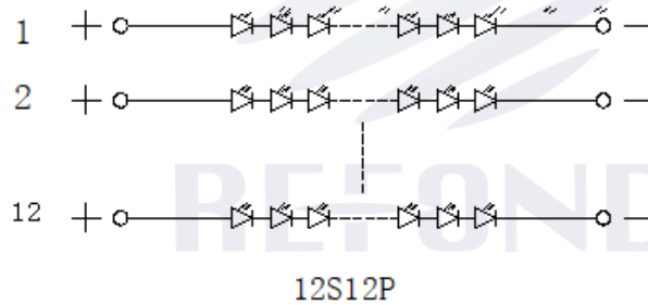
Fig.1-3 Polarity 极性
