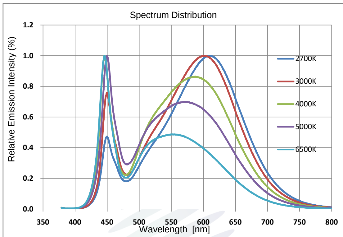
Fig 1-13 Spectrum Distribution 光谱分布特性曲线
