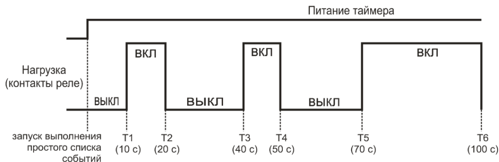
Рисунок 3.6 – Включение нагрузки на примере простого режима работы
