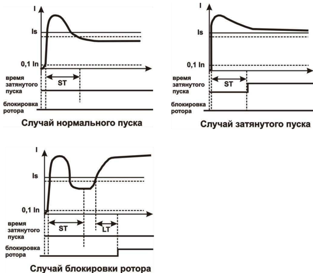
Рисунок 1.4 - Затянутый пуск и блокировка ротора
