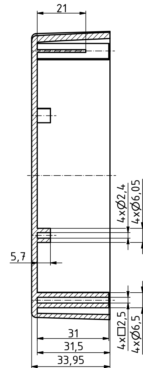
C-C ( 1 : 1 )
