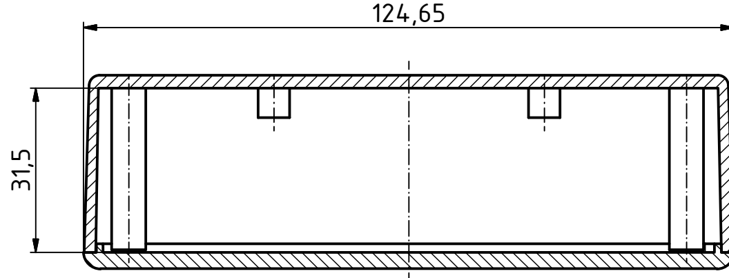
A-A ( 1 : 1 )
