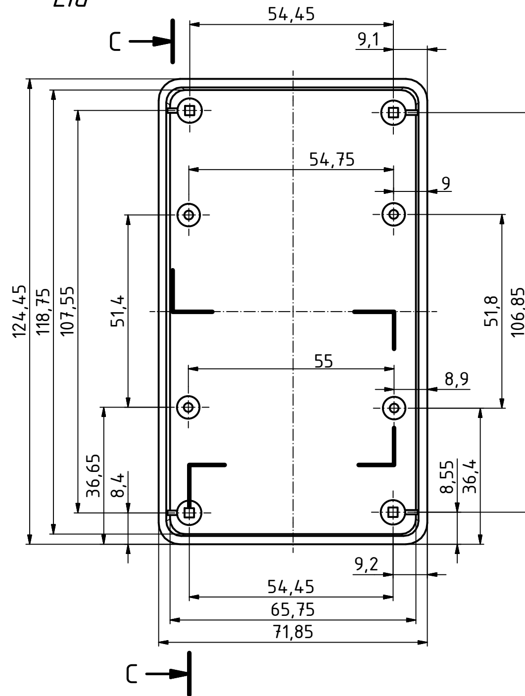
Oberteil/ Lid
