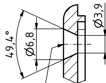
Z ( 2 : 1 )
