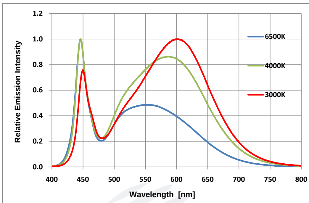
Fig 1-13 Spectrum Distribution光譜分布特性曲線
