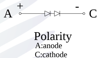
Fig.1-4 Polarity 极性
