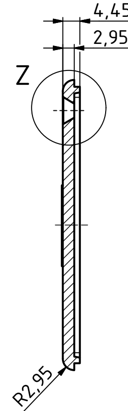
B-B ( 1 : 1 )
