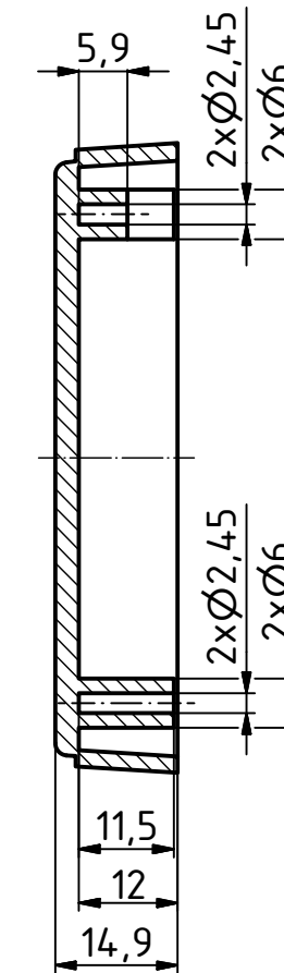
C -C ( 1 : 1 )
