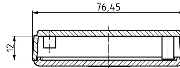
A-A ( 1 : 1 )
