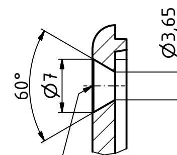
Z ( 2 : 1 )
