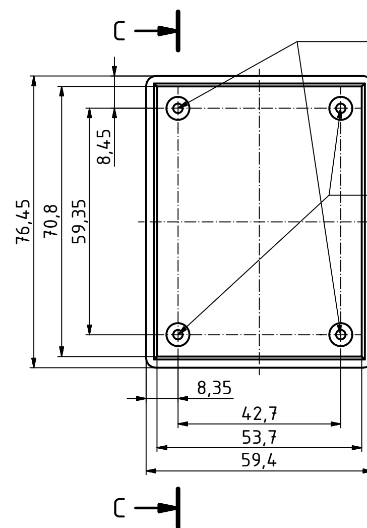
Oberteil/ Lid
