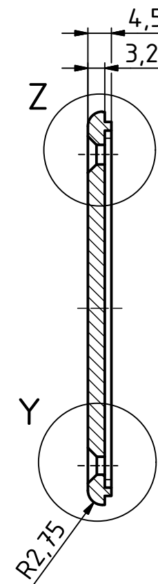
B-B ( 1 : 1 )
