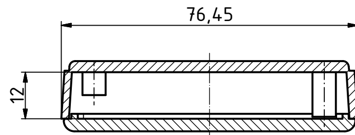
A-A ( 1 : 1 )
