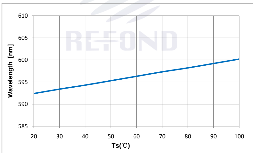
Fig 1-11 Wavelength Vs. Pin Temperature 波长与管脚温度特性曲线
