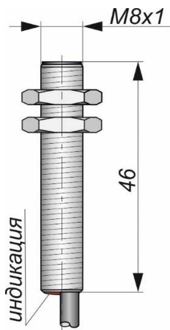
Габаритный чертеж
