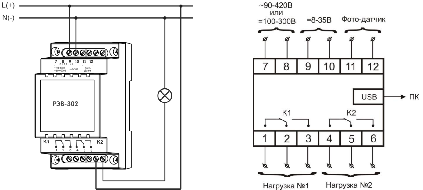
Рисунок 2.1 - Электрические соединения РЭВ-302
