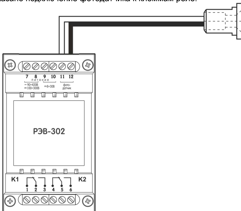
Рисунок 1.3 - Подключение фотодатчика к РЭВ-302
