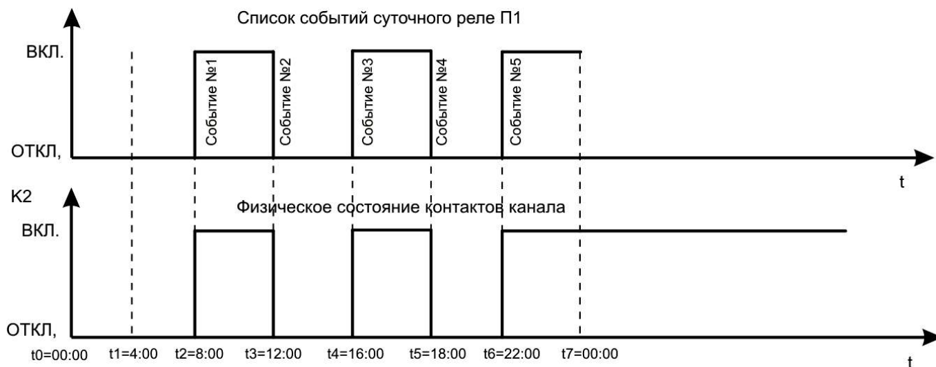
Рисунок 2.7 - Режим однократного выполнения списка таймеров на примере суточного реле времени
